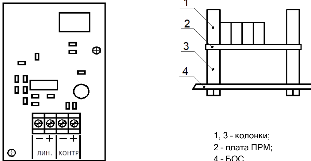
а) Общий вид платы ПРМ
